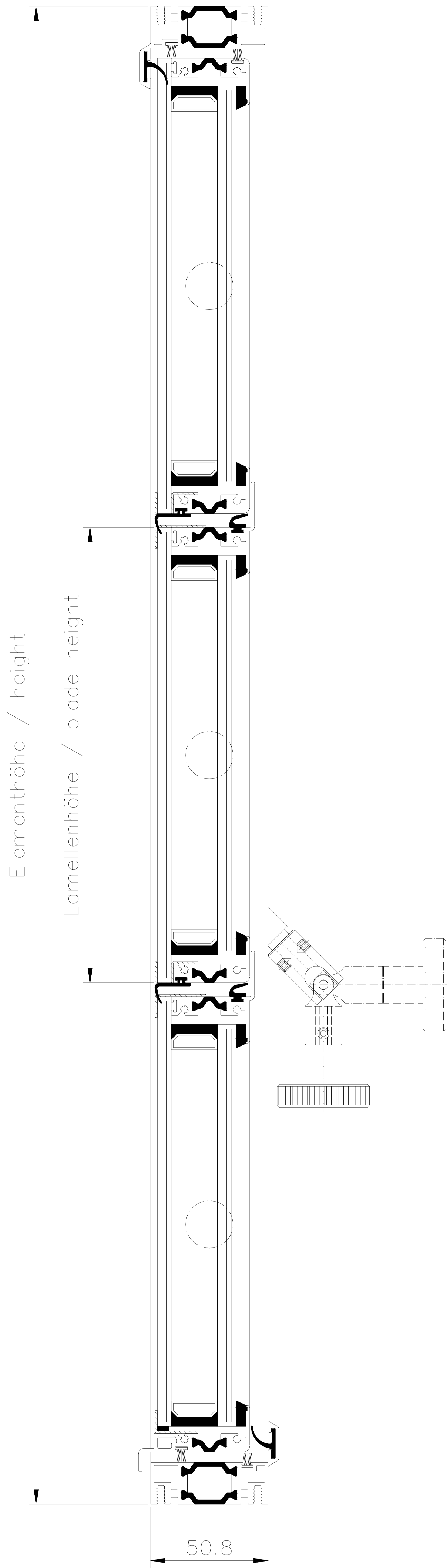
Für 34er Glas mit 6er Glas Außen / For 34mm glazing, 6mm outer pane
